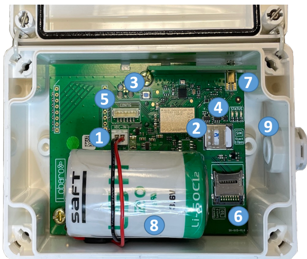
Abbildung 1: Geräte Komponenten
